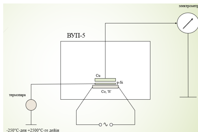
1-сурет. Күн түрлендіргіштерінің бетінің электрлік қасиеттерін алуға сұлбасы
